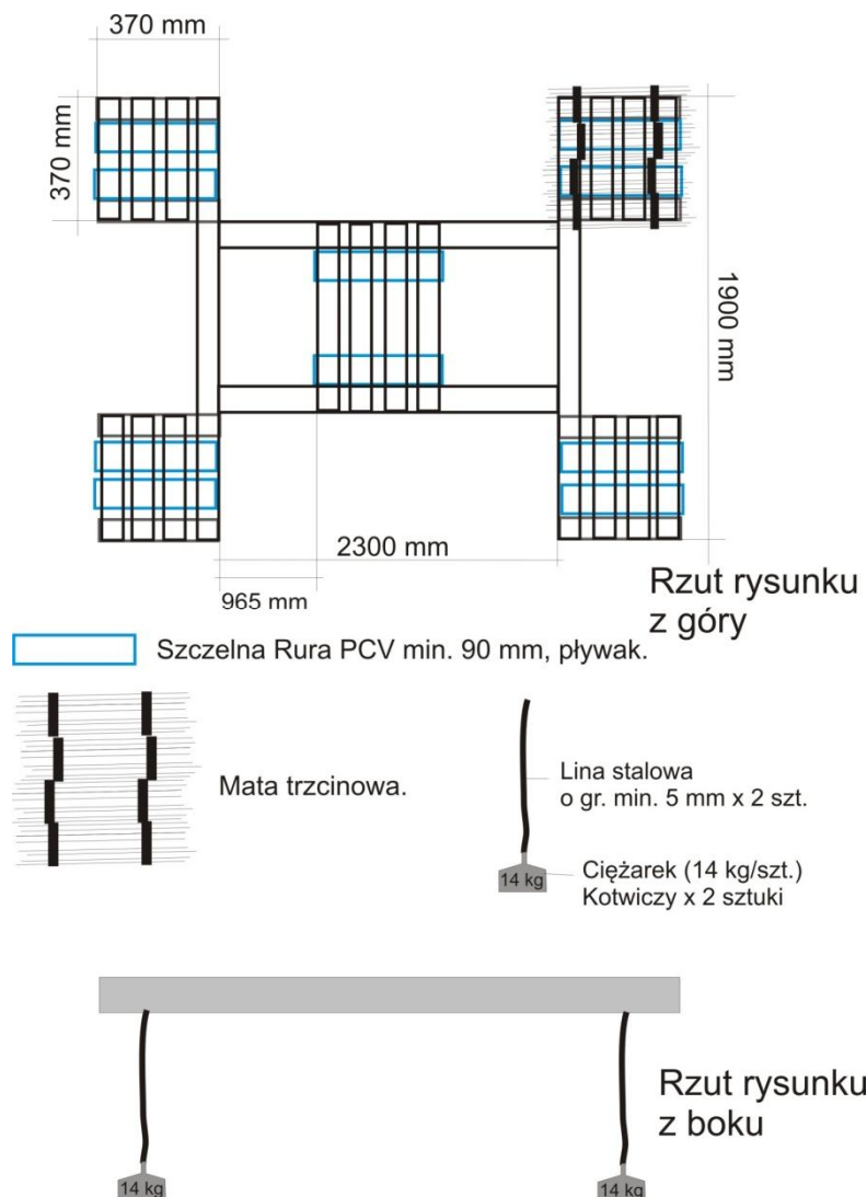
Rys. 1: Schemat platformy dla rybitwy czarnej.
